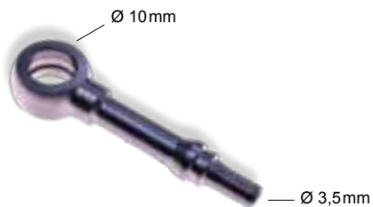
00040 Art.-Nr. 23-10004030
