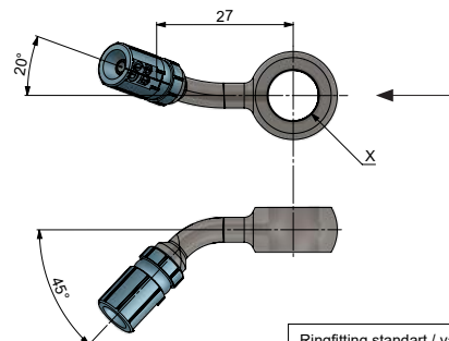
Ausrichtung: Ringfitting in Pfeilrichtung halten Ringfitting standart / vario 45° seitlich / 20° rechts gebogen
