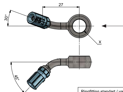
Ausrichtung: Ringfitting in Pfeilrichtung halten Ringfitting standart / vario 45° seitlich / 30° rechts gebogen
