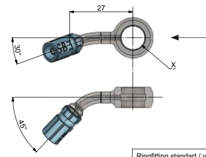
Ausrichtung: Ringfitting in Pfeilrichtung halten Ringfitting standart / vario 45° seitlich / 30° links gebogen
