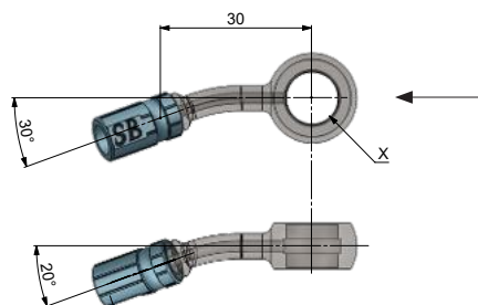
Ausrichtung: Ringfitting in Pfeilrichtung halten Ringfitting standart / vario 20° seitlich / 30° links gebogen
