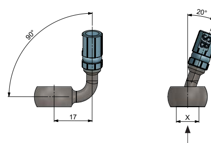
Ausrichtung: Ringfitting in Pfeilrichtung halten Ringfitting standart / vario 90° seitlich / 20° rechts gebogen
