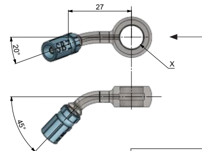
Ausrichtung: Ringfitting in Pfeilrichtung halten Ringfitting standart / vario 45° seitlich / 20° links gebogen
